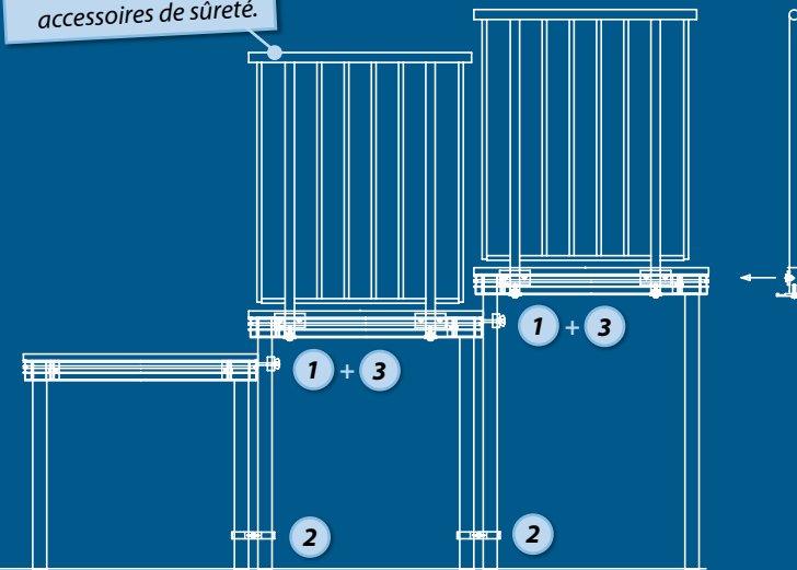
Version gradin avec accessoires de sûreté.
